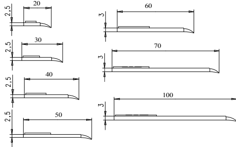
1/5 Flachleisten mit langer Weichlippe
