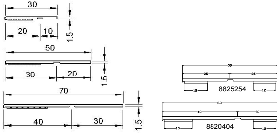
1/2 Knickwinkel und Flachleisten auf Rolle
