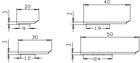
1/6 Flachleisten mit kurzer Weichlippe
