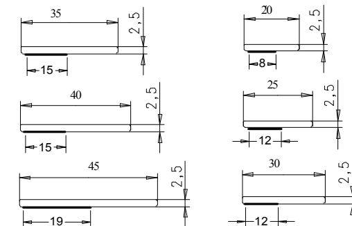
1/09 Flachleisten 2,5mm stark
