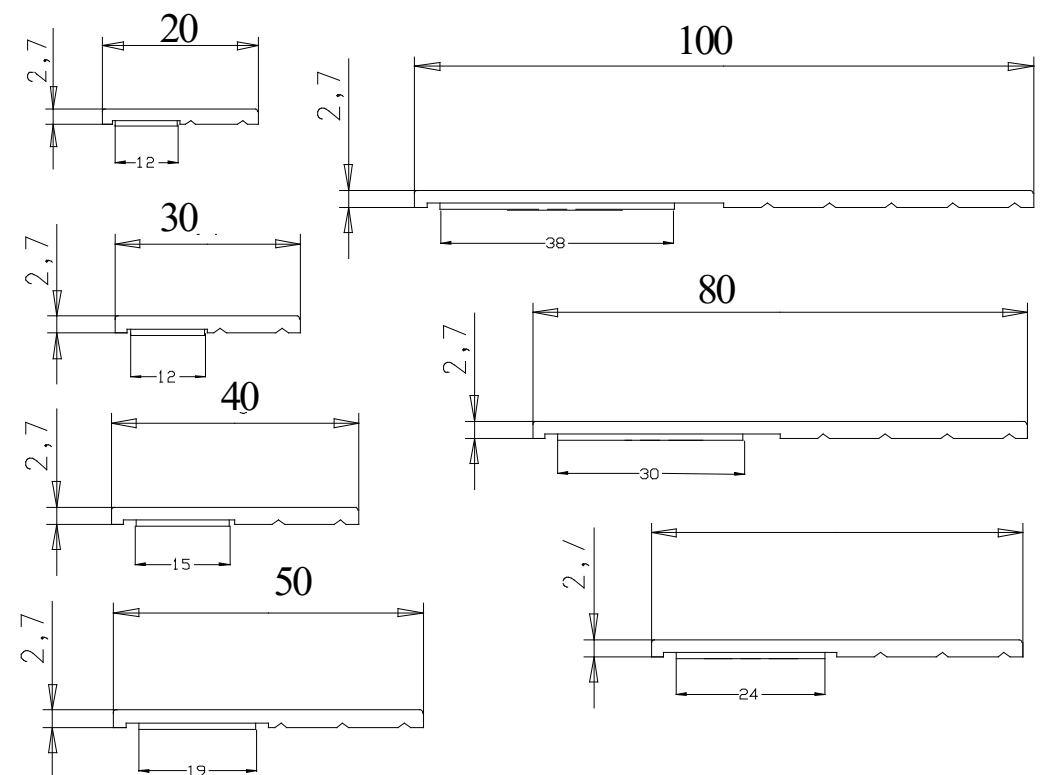
1/7 Flachleisten mit SKS und Abdecknase
