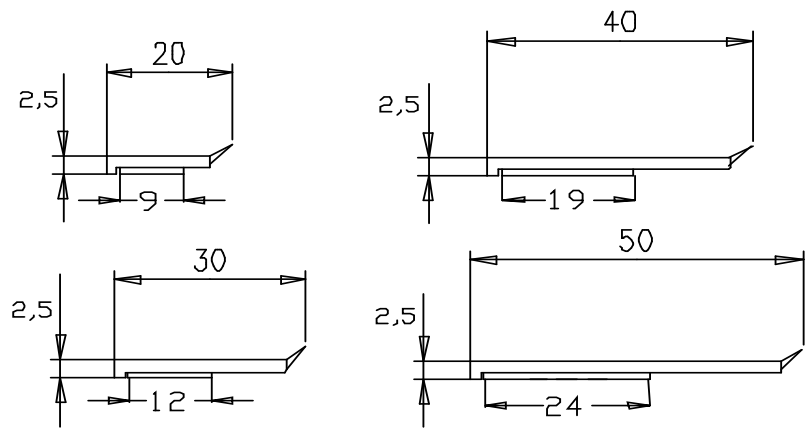
1/6 Flachleisten mit kurzer Weichlippe
