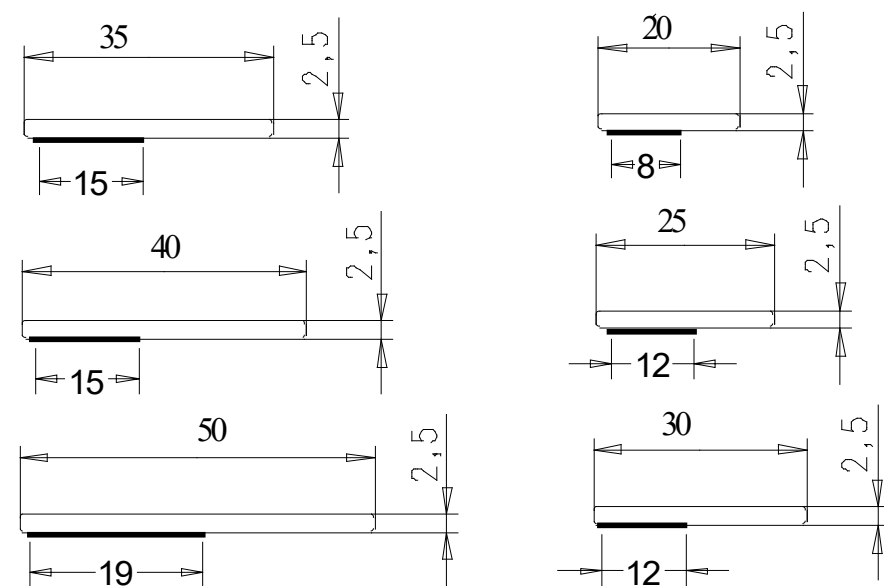
1/9 Flachleisten 2,5mm stark
