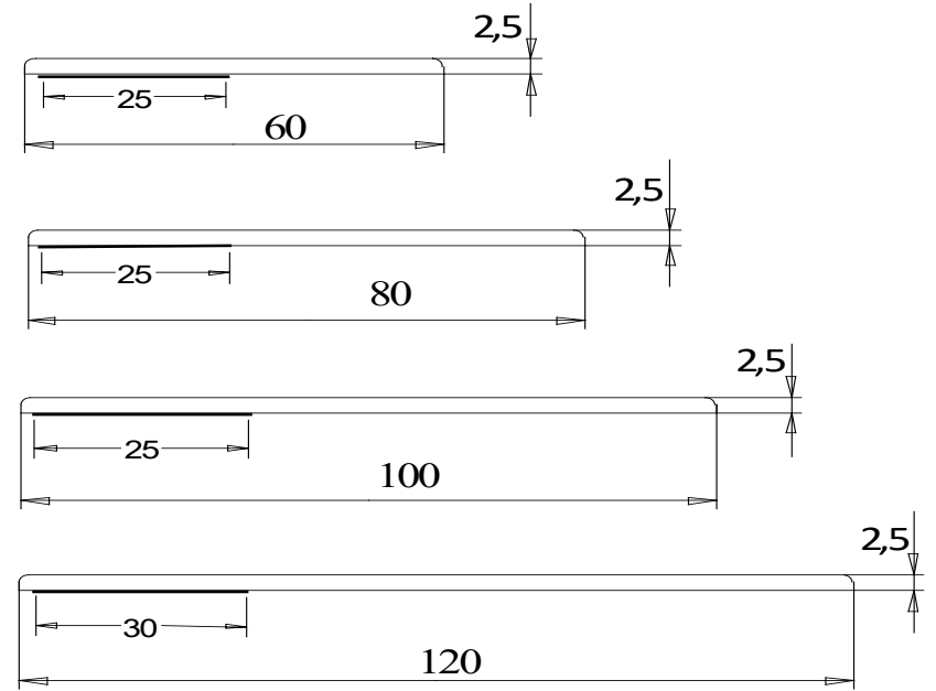
1/8 Flachleisten 2,5mm stark
