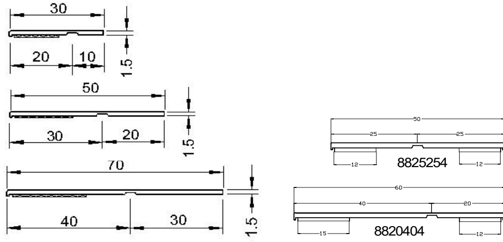
1/2 Knickwinkel und Flachleisten auf Rolle
