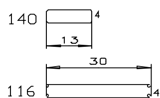
1/11 Flachleisten 4mm stark
